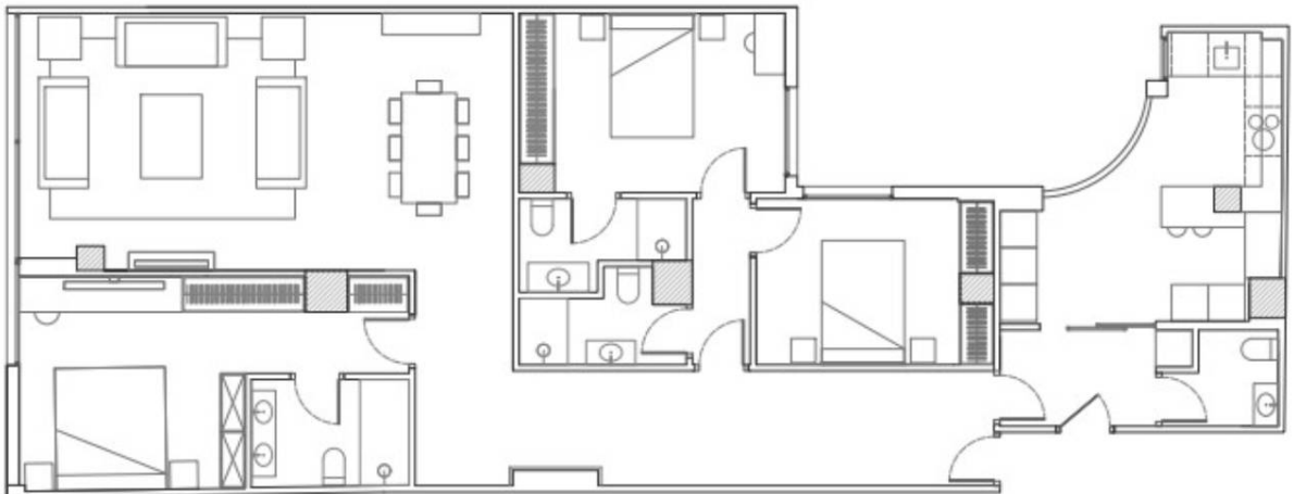
PLANO DISTRIBUCIÓN
